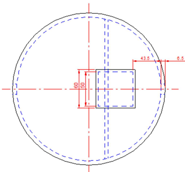
Bovenaanzicht
