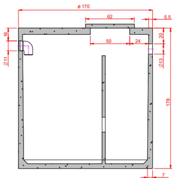
Doorsnede
