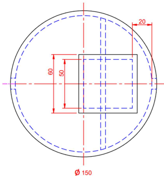
Bovenaanzicht
