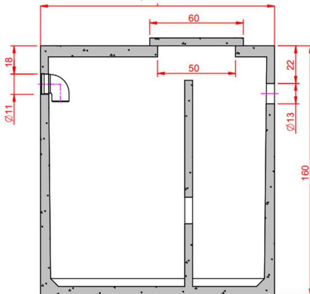
Doorsnede
