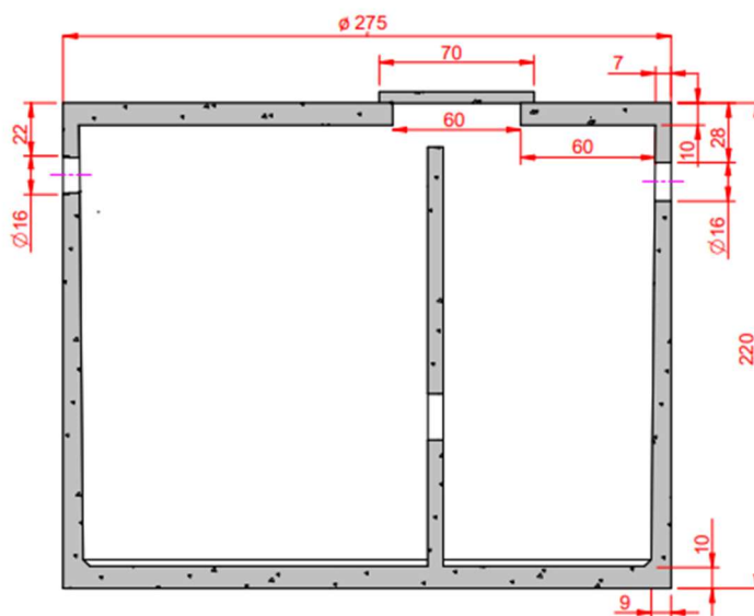
Doorsnede
