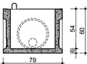
DOORSNEDE COUPE
