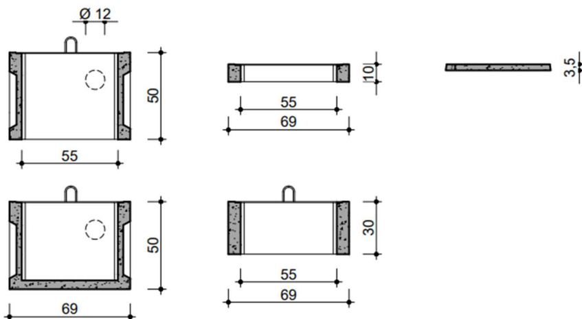
DOORSNEDE COUPE
