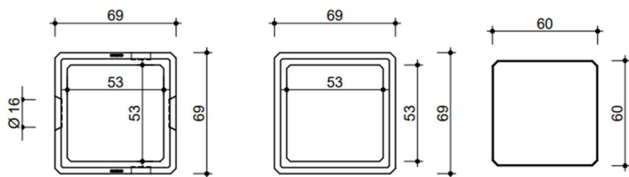
BOVENAANZICHT VUE DE DESSUS
