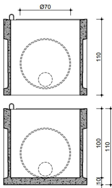
DOORSNEDE COUPE
