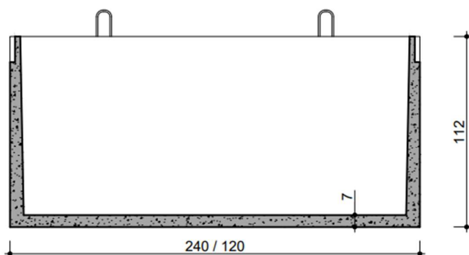
DOORSNEDE COUPE
