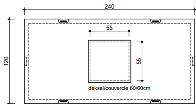
BOVENAANZICHT VUE DE DESSUS
