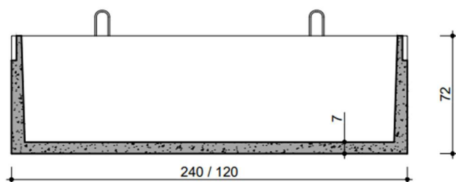
DOORSNEDE COUPE
